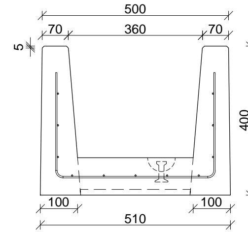
Snit A-A
